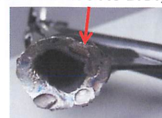
DETALHE DO CORDÃO DE SOLDA JUNTO AO BRAÇO
