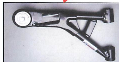
BRAÇO SUPERIOR DA SUSPENSÃO DIANTEIRA DIRETA
