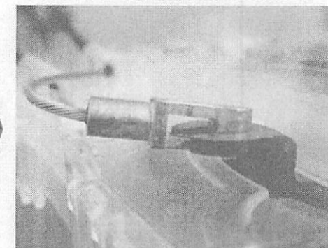
CABO DE ACIONAMENTO DA MAÇANETA INTERNA DESLOCADO JUNTO A TRAVA DA PORTA
