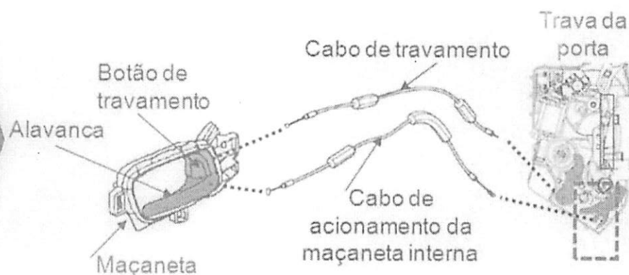
SISTEMA DE TRAVAMENTO DAS PORTAS DIANTEIRAS
