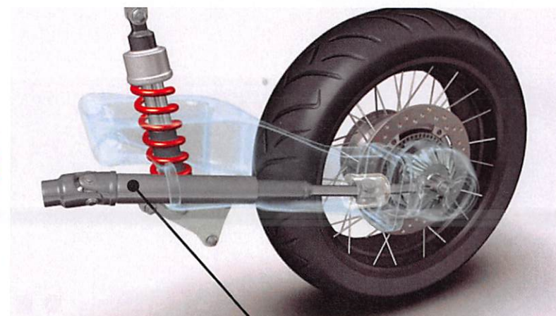
Visão Interna do Sistema de Transmissão Final
