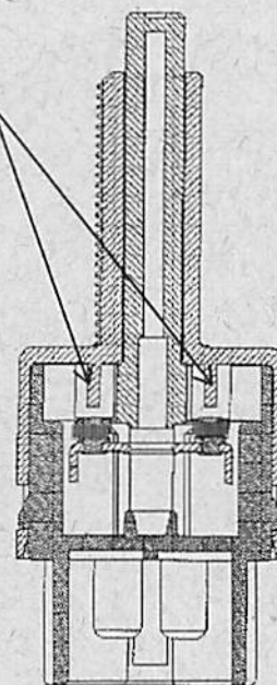
Figura 2 – Interruptor da luz de freio, detalhe dos terminais onde ocorre o isolamento elétrico.
